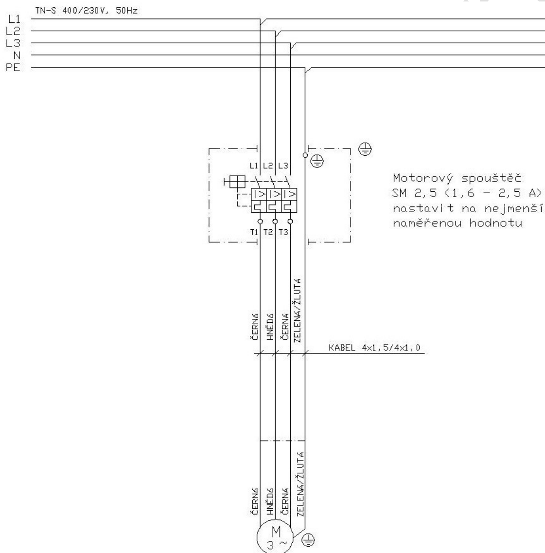
Schéma zapojení motorového spouštěče s čerpacím agregátem obr. 8
